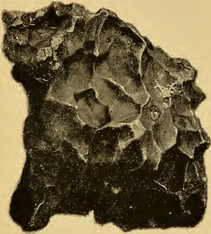
FIG. 95.—Meteorite.
